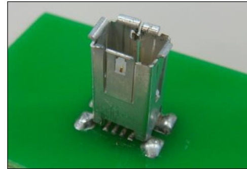
Tyco Electronics社製 IMIコネクタ バーチカルタイプ
